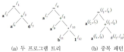
그림 2. 두 프로그램 트리의 중복 패턴
