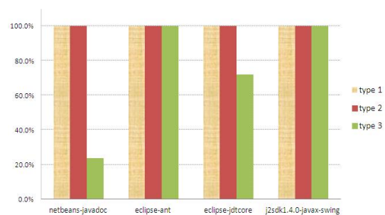
그림 7. 파라미터 HoleMassLimit=25로 실험한 코드클론 유형별 탐지성
