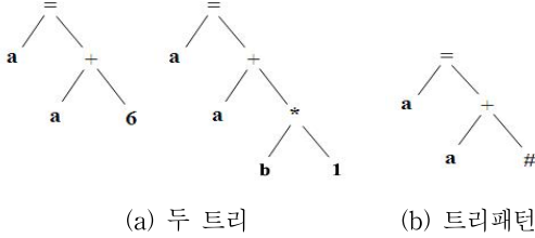
그림 1. 두 트리의 트리 패턴
