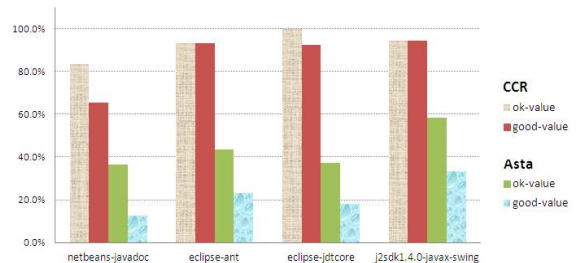
그림 10. CCR과 Asta의 ok-value와 good-value 비율
