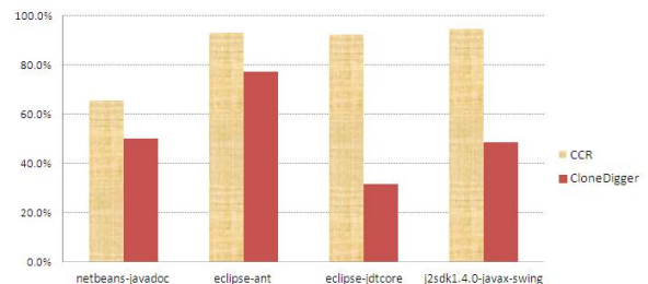
그림 11. CCR과 CloneDigger의 탐지성
