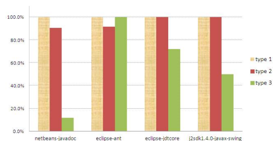
그림 5. 파라미터 HoleMassLimit=10으로 실험한 코드클론 유형별 탐지성
